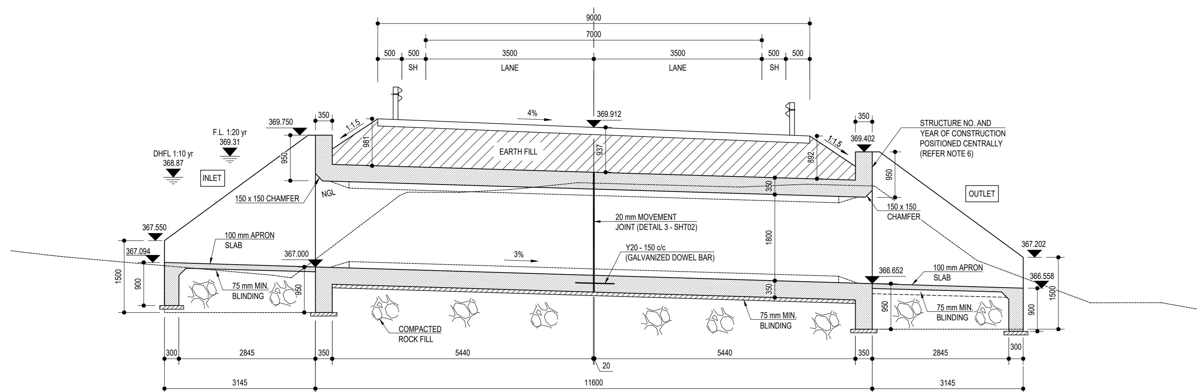
LONGITUDINAL SECTION A - A 1:50
